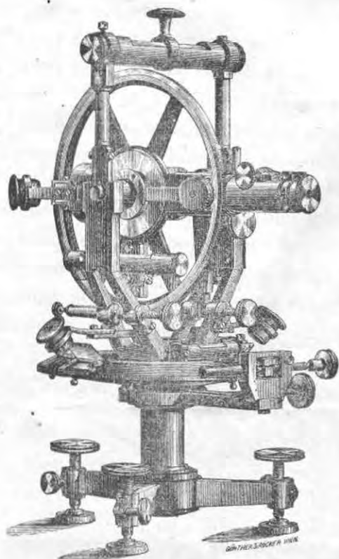
Fig. 2. Nr. 110 ( \frac{1}{3} tamaño natural).
