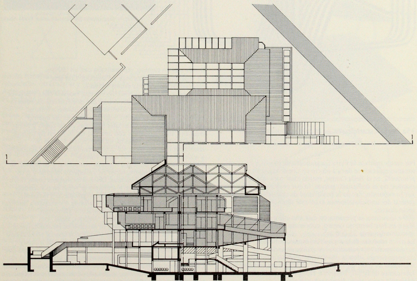
CORTE 1-1
