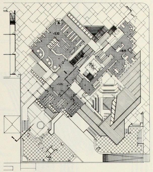
PLANTA NIVELES +632 +815
